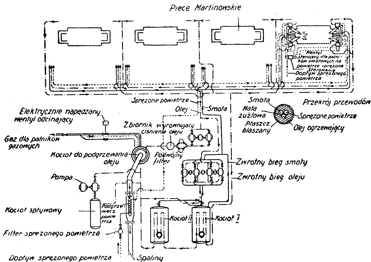
Urządzenia karburacyjne na smołę dla 4 pieców martenowskich.
